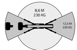
REDUZIERTE ABSTÜTZFLÄCHE
